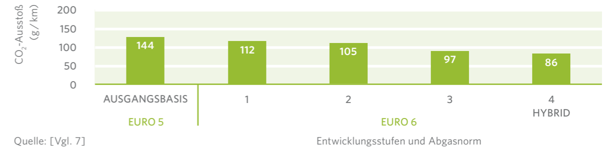
Abbildung 3: CO 2 -Reduzierungspotential von dieselbetriebenen Motoren durch Downsizing und Hybridtechnologie
