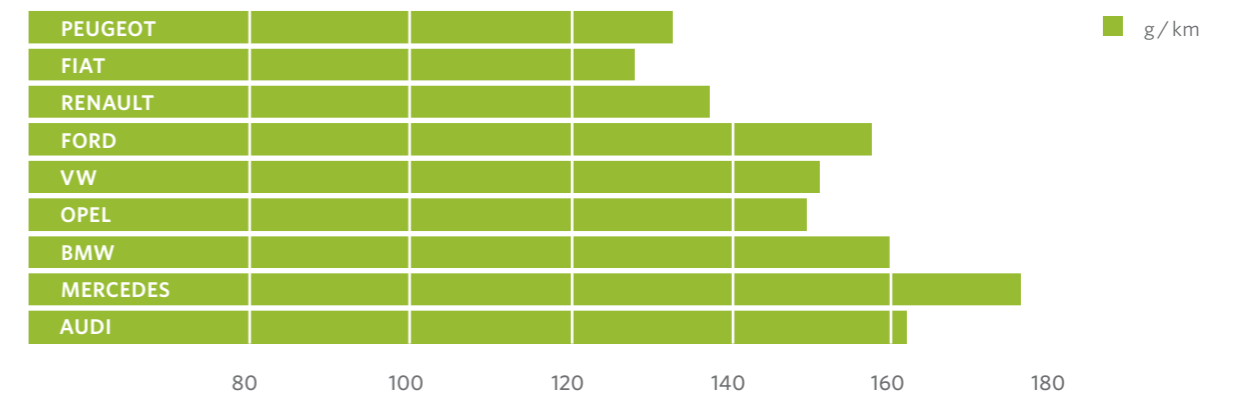
Abbildung 1: Durchschnittlicher CO 2 -Ausstoß deutscher Pkw-Neuzulassungen
