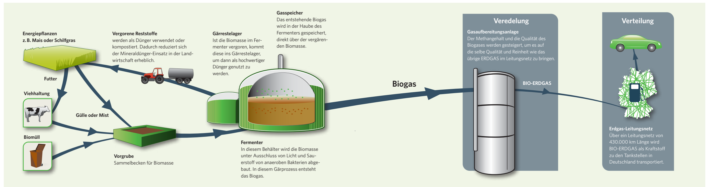
Abbildung 9: Schema einer zweistufigen Biogasanlage mit Gasaufbereitung
