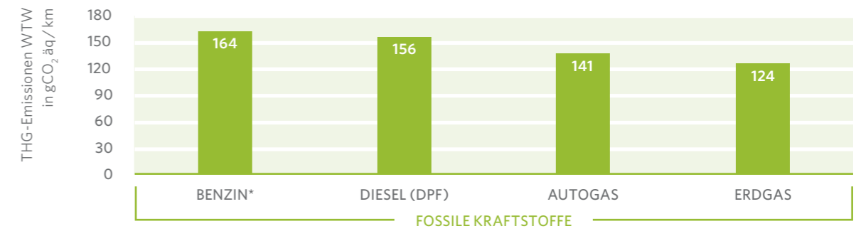
Abbildung 4: Treibhausgasemissionen unterschiedlicher fossiler Kraftstoffe
