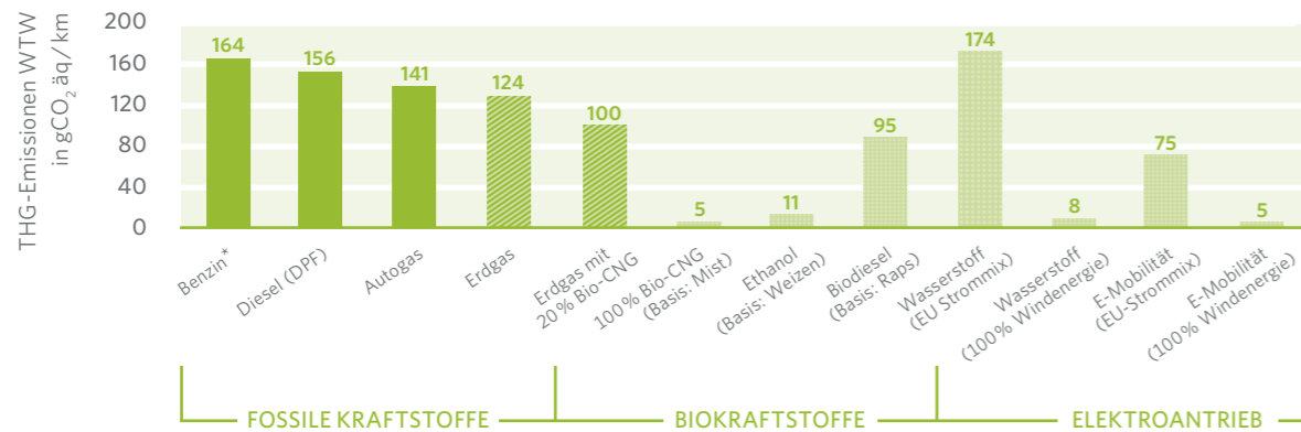
Abbildung 11: Treibhausgasemissionen unterschiedlicher Kraftstoffe
