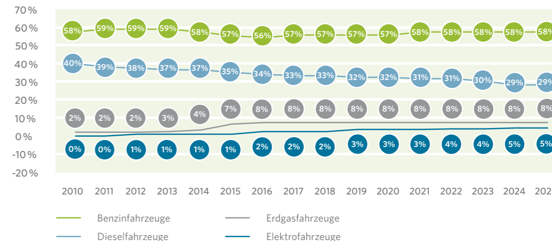
Abbildung 16: Potentielle Marktentwicklung von Benzin-, Diesel-, Erdgas- und Elektrofahrzeugen in Deutschland (2010 bis 2025)
