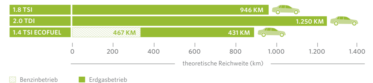
Abbildung 7: Der VW Passat mit unterschiedlichen Reichweiten im Benzin-, Diesel- und Erdgasbetrieb
