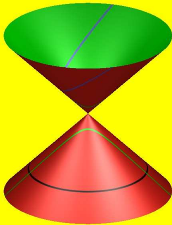
Schnitte eines Kegels mit Ebenen: Hyperbel, Ellipse und Parabel
