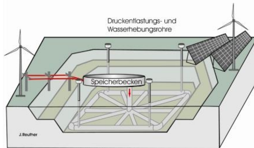
Verfüllter Tagebau mit Pumpspeicher
