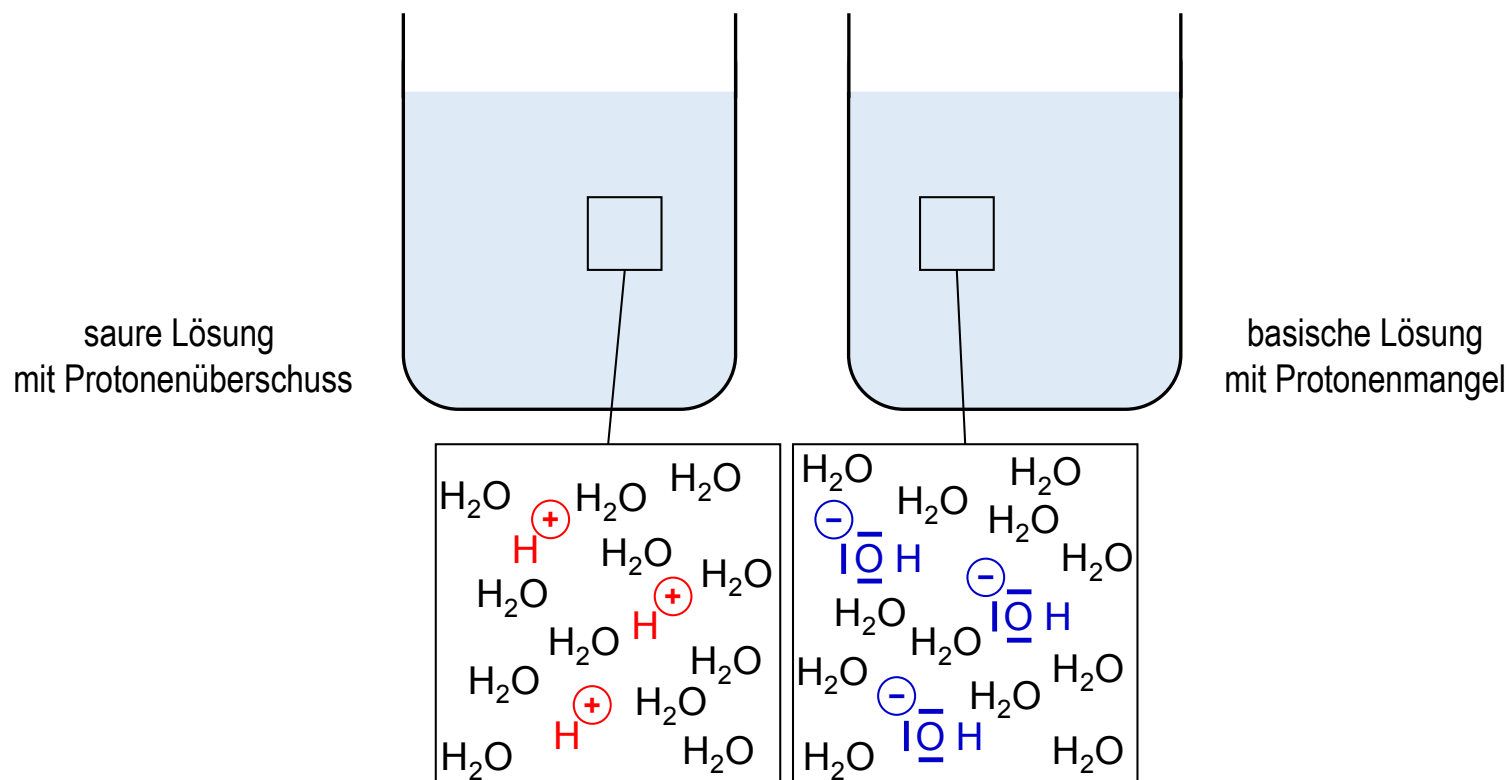
Bild 9: Saure und basische Lösung
