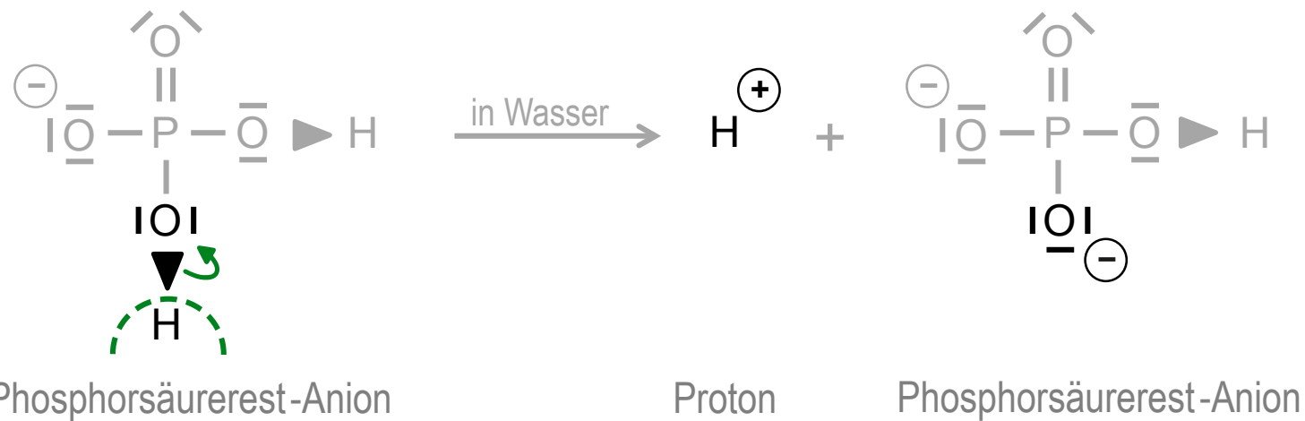
Bild 11: Dissoziation eines zweiten Protons
