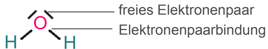
Bild 14: Bindende und freie Elektronenpaare im Wassermolekül
