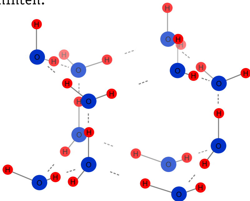
Bild 15: Anordnung der Wassermoleküle im Eis
