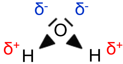
Bild 29: Partialladungen im Wassermolekül
