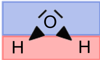
Bild 31: Pole mit entgegengesetzter Ladung im Wassermolekül
