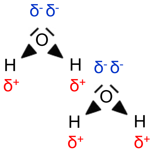
Bild 10: Zwei Wassermoleküle
