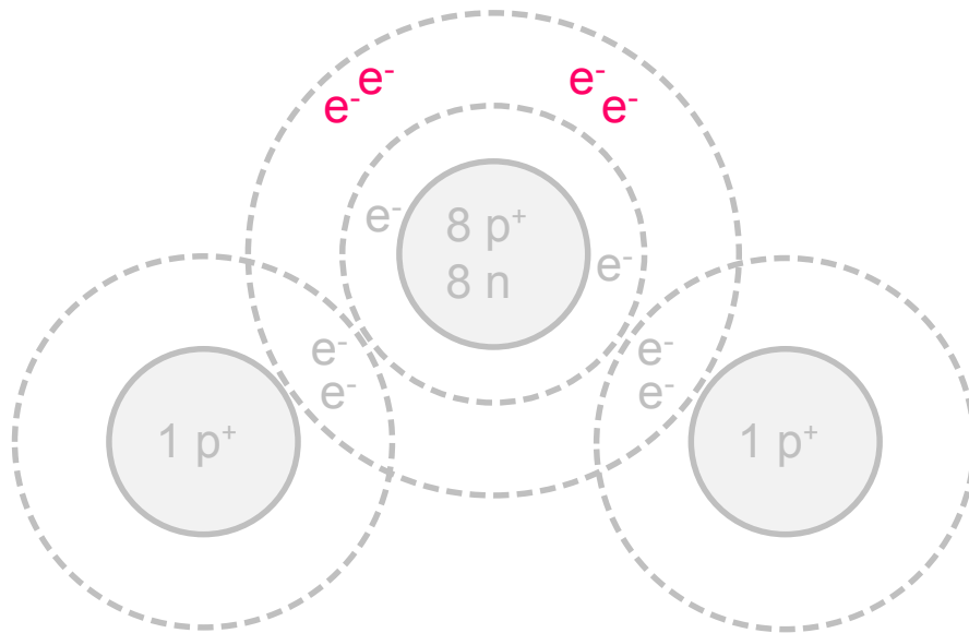
Sauerstoffatom
