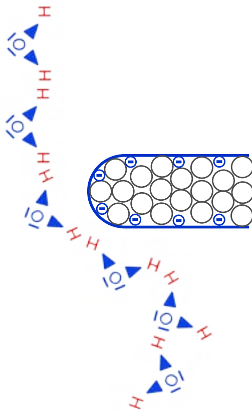
Bild 33: Wassermoleküle, die von einem elektrostatisch geladenen Stab angezogen werden
