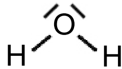
Bild 3: Strukturformel eines Wassermoleküls
