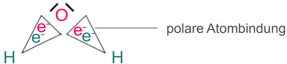
Bild 25: Polare Atombindungen im Wassermolekül
