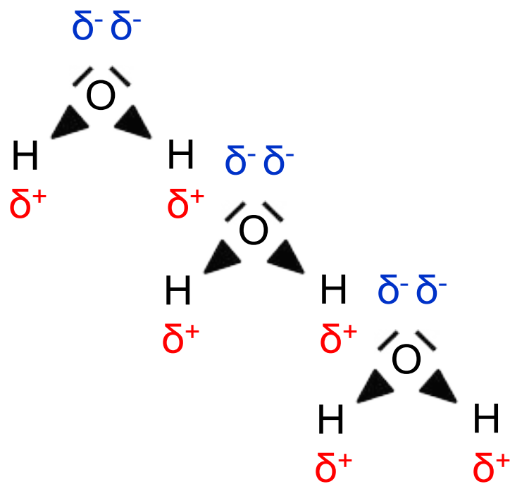
Bild 12: Drei Wassermoleküle
