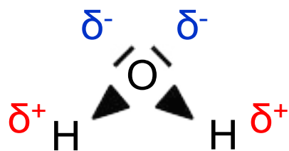
Bild 9: Partialladungen im Wassermolekül
