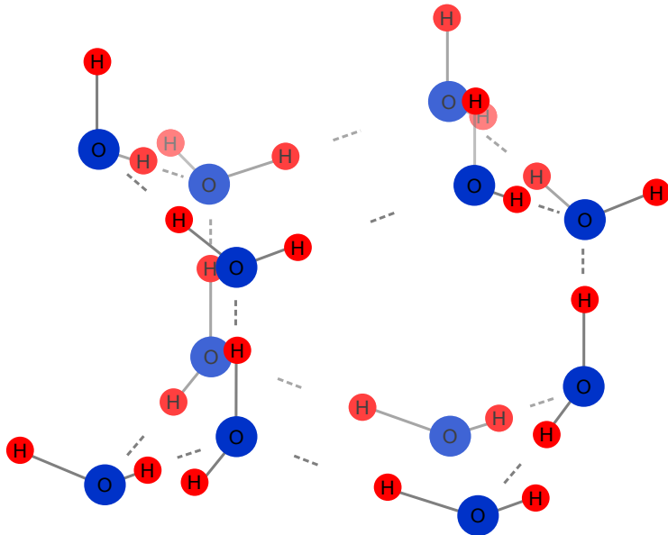
Bild 19: Anordnung der Wassermoleküle im Eis
