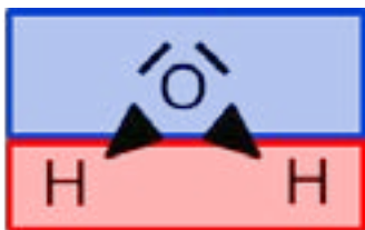
Bild 4: Pole mit entgegengesetzter Ladung im Wassermolekül
