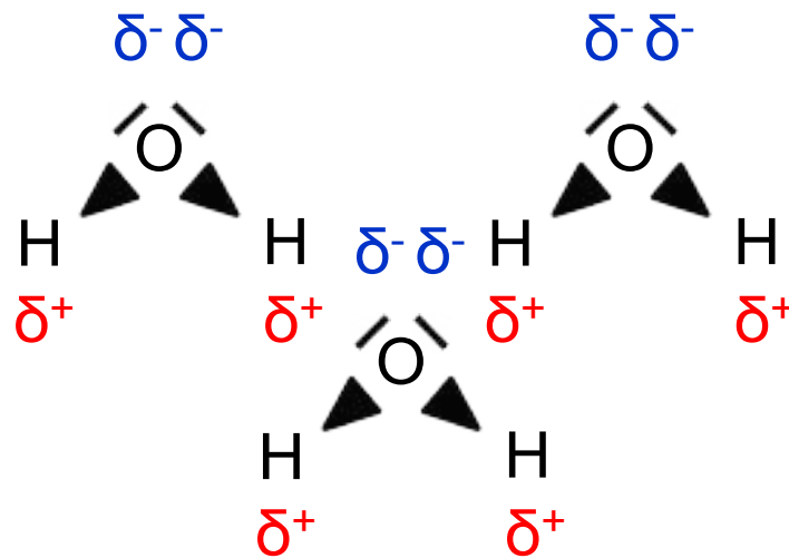
Bild 11: Drei Wassermoleküle
