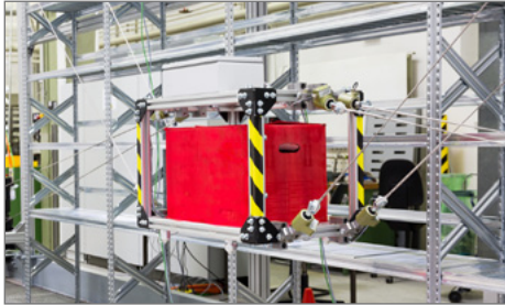
Seilroboter in einem Hochregallager. © Lehrstuhl Rechnereinsatz in der Konstruktion
