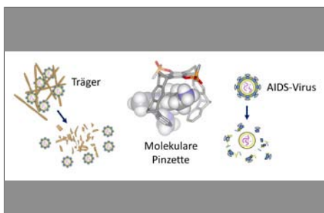
So funktioniert die molekulare Pinzette bei AIDS. © UDE/Thomas Schrader
