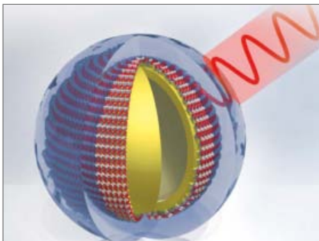
Ein Edelmetallnanopartikel für oberflächenverstärkte Raman-Spektroskopie. © Sebastian Schlücker/UDE
